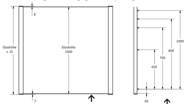
Glas-Abmessungen und Befestigungsabstände Top Montage
